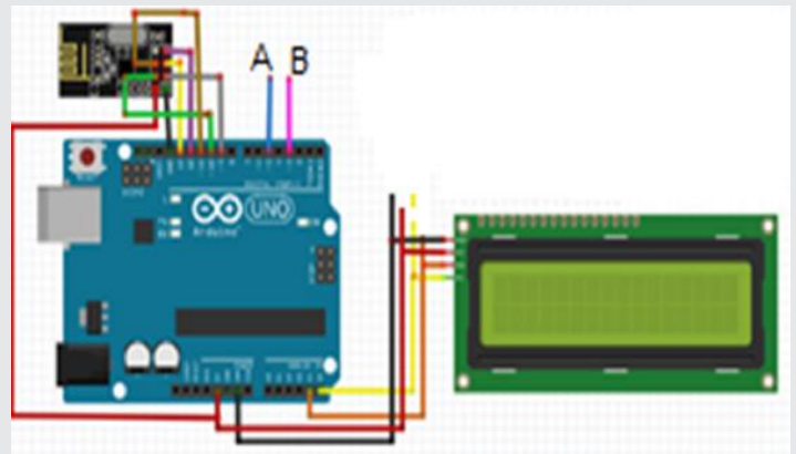
Figura 7. Transmisor maestro.
