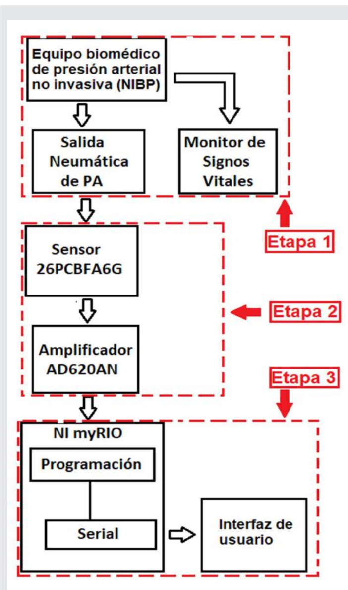
Figura 1. Sistema de evaluación de algoritmos de presión arterial.
