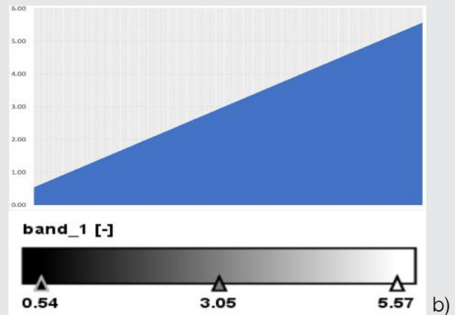
Figura 6. LAI: a) Fecha: 05-10-2018, b) Fecha: 01-08-2019.
